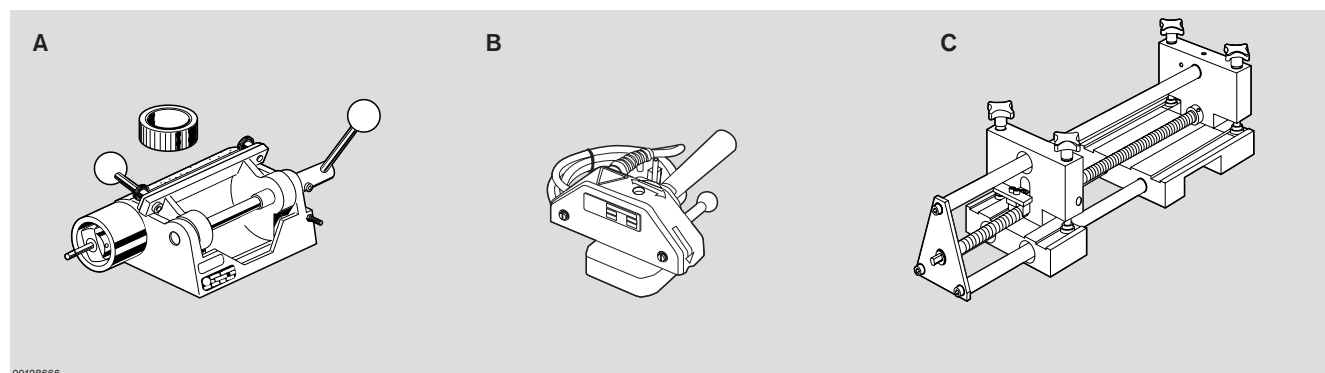
Gurtmontage-Werkzeugsatz Belt mounting tool kit Kit d'outillage de montage de courroies
