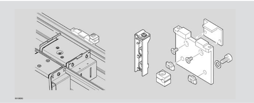
Beispiel: EQ 1/TR mit Anschlagleiste Example: EQ 1/TR with stop rail Exemple : EQ 1/TR avec barre de butée
