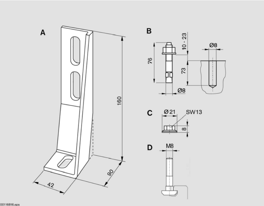
Fundamentwinkel Foundation bracket Equerre de fondation
