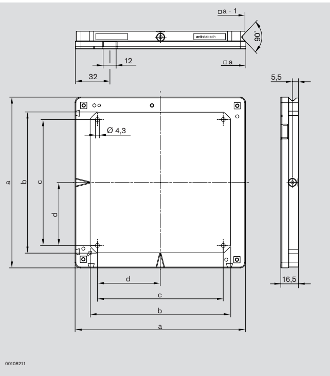
Werkstückträger WT 1/S Workpiece pallet Palette porte-pièces
