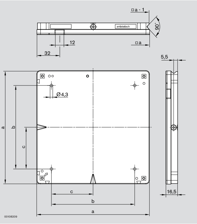
Werkstückträger WT 1/K Workpiece pallet Palette porte-pièces
