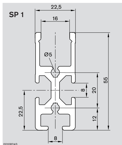
Streckenprofil SP 1 Section profile Profilé de section
